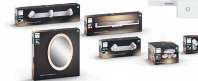
Adore Hue zápusťné svítidlo chrom 3407411P7 ↓ 70–75 ↔ 94 ↗ 94 mm 1×5 W, GU10, 350 lm max. Dimmer Switch není v balení
